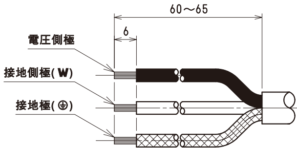
☆電線加工寸法
