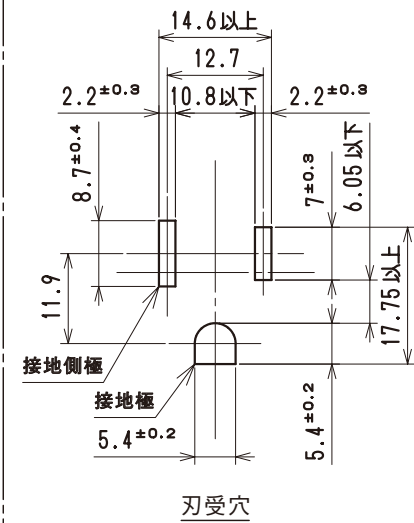
極配置寸法
